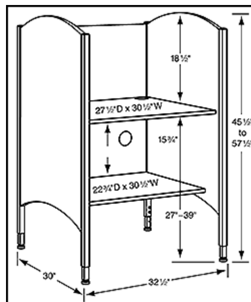
Kiosk Dimensions
